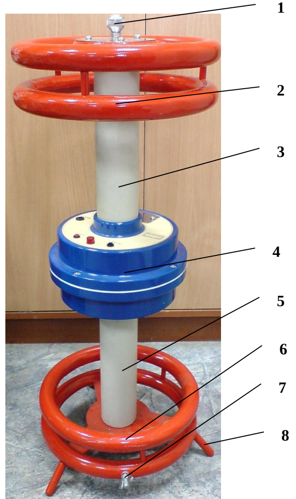
Рисунок 2. Блок высоковольтный РД140-БВ. Вид общий
