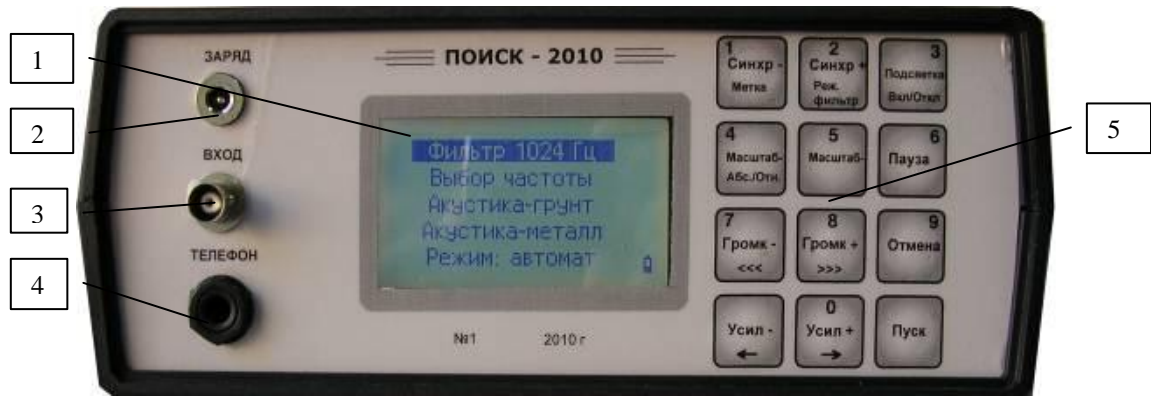
Рисунок 9. Приемник «ПОИСК-2006м». Панель лицевая.
