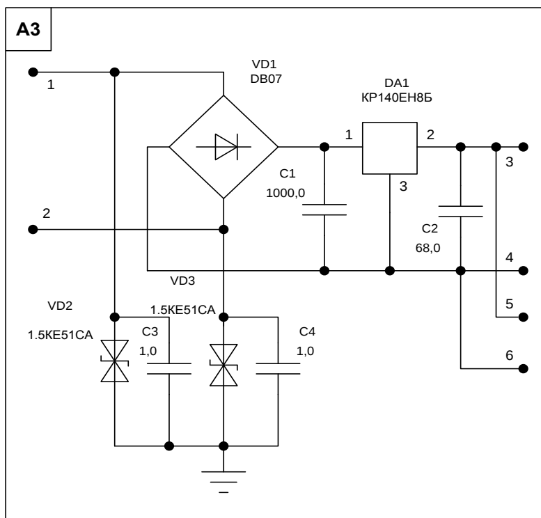
Рис. 2. Электролаборатория КАЭЛ-5. Блок управления. Плата A3. Стабилизатор напряжения. Схема электрическая принципиальная
