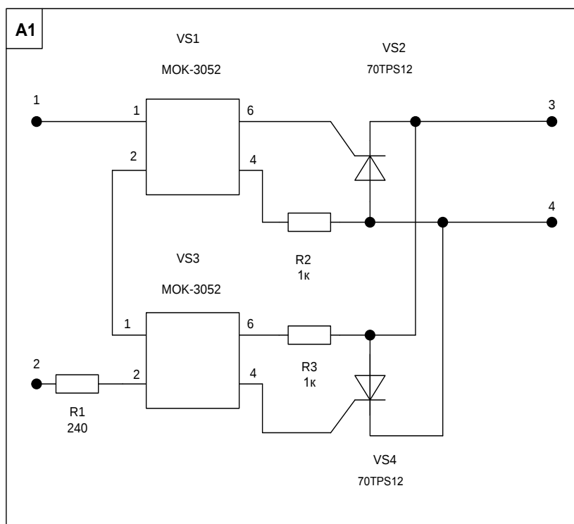
Рис. 1. Электролаборатория КАЭЛ-5. Блок управления. Плата A1. Тиристорный регулятор. Схема электрическая принципиальная
