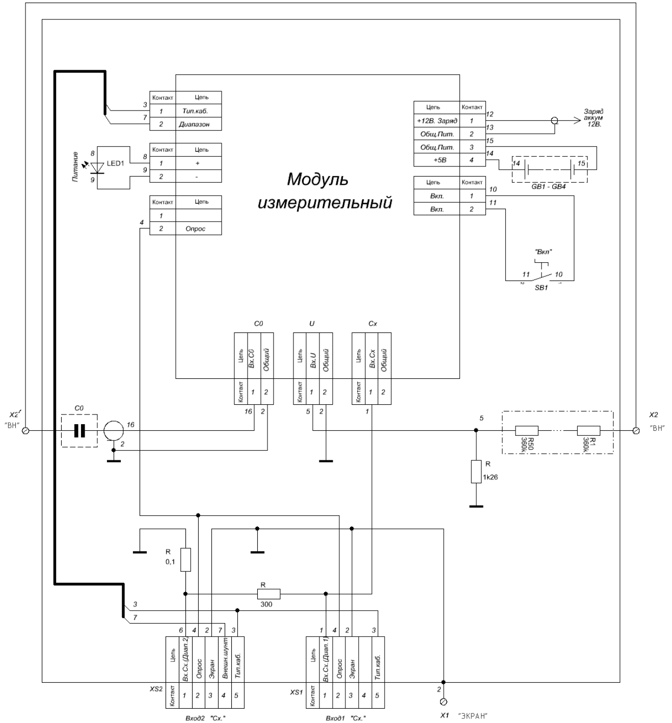
Рис.1 Блок высоковольтный ИПИ-10-БВ. Схема электрическая принципиальная.
