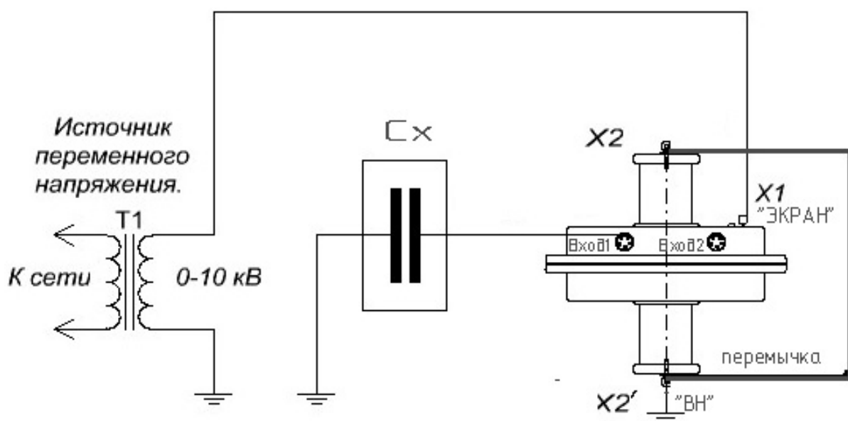
Рисунок 5. «Перевернутая» схема измерений
