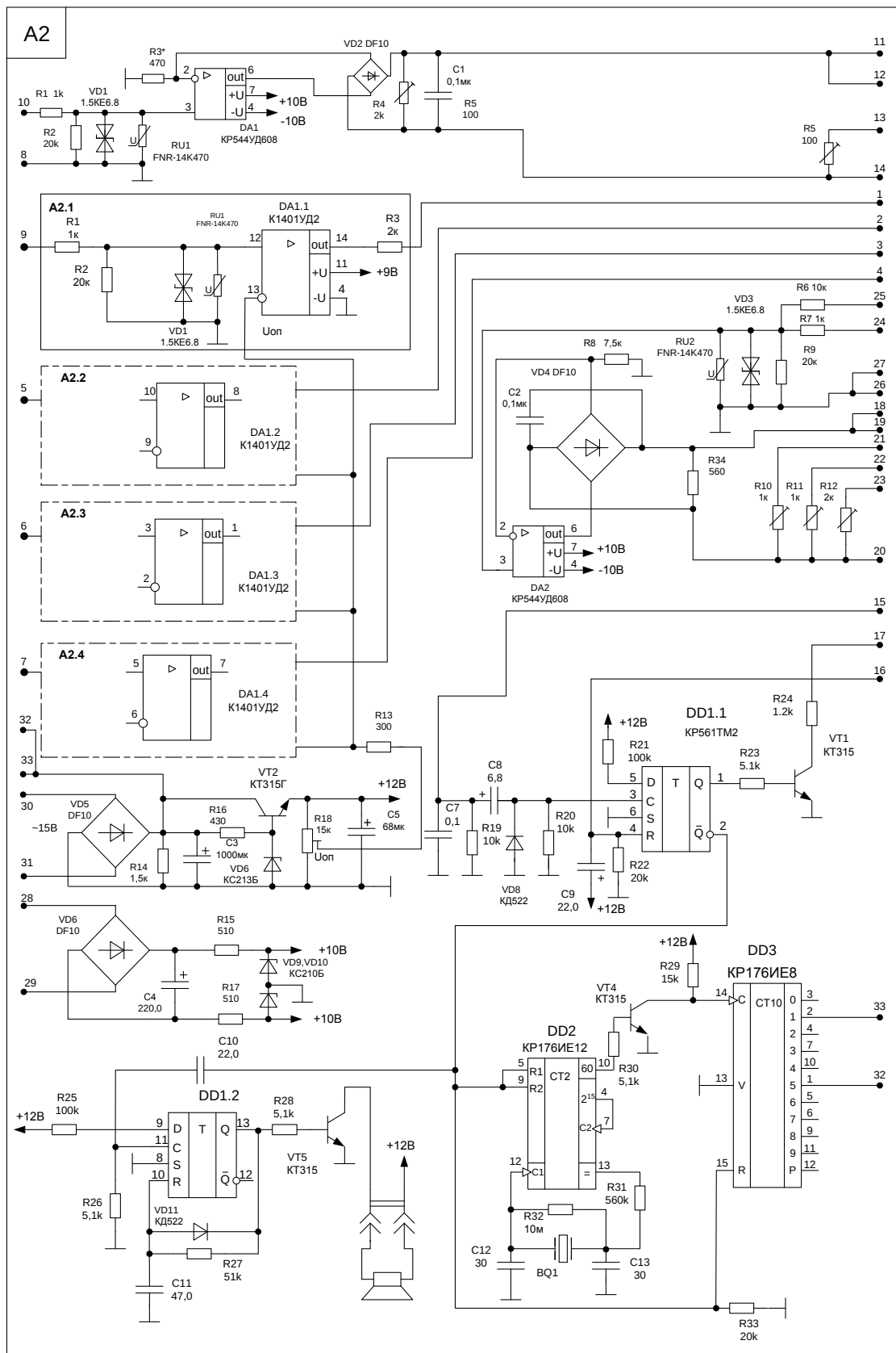
Приложение 4 Стенд высоковольтный стационарный СВС-50 Блок управления. Узел управления 2. Схема электрическая принципиальная
