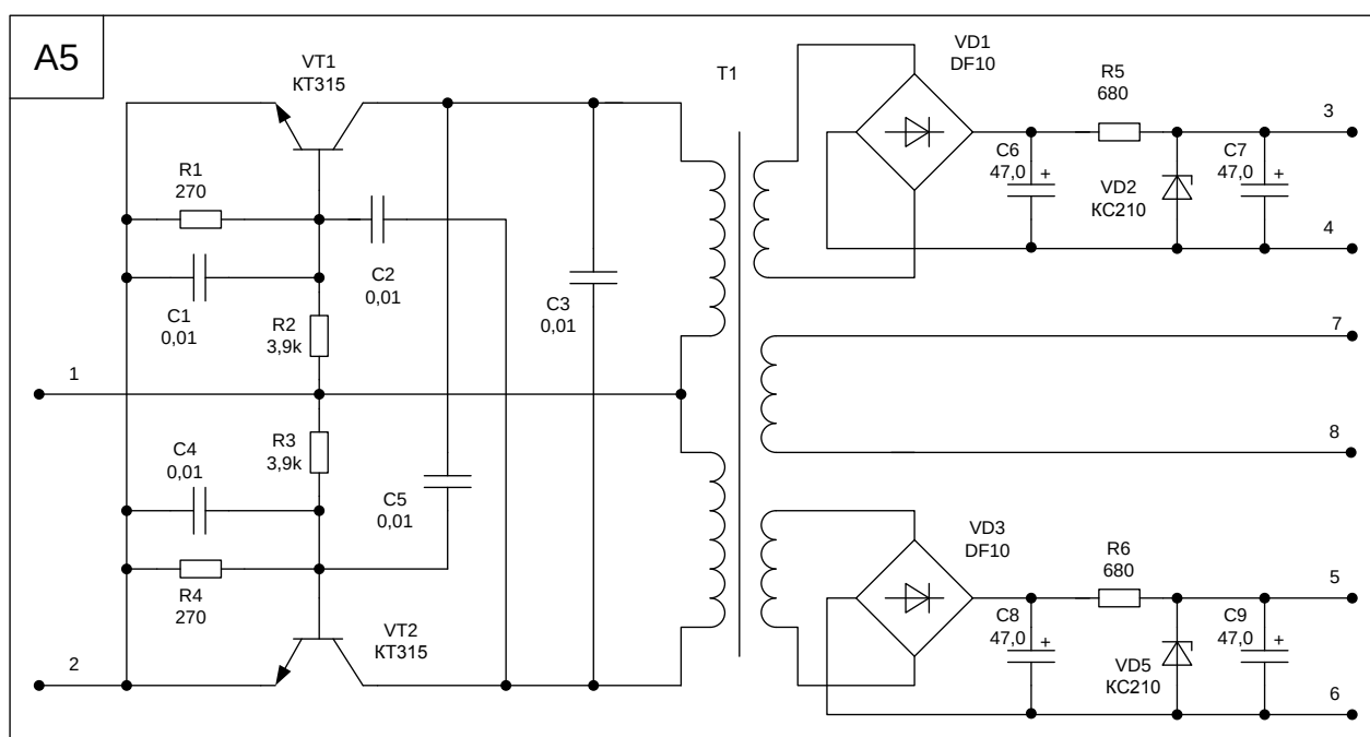
Рис.3. Схема подключения блока БВИ-50-1 при регулировке порога зажигания светодиодов
