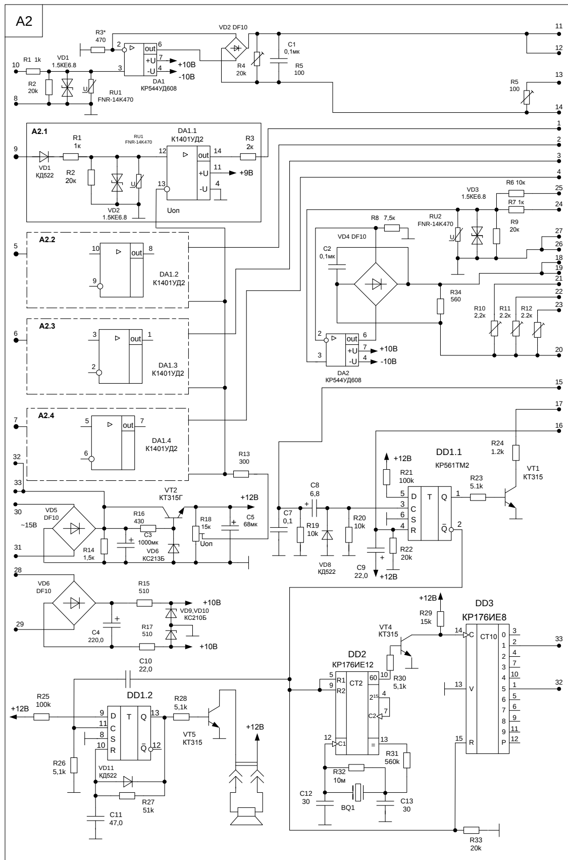
Приложение 4 Стен высоковольтный стационарный SVC-100 Блок управления. Узел управления 2. Схема электрическая принципиальная
